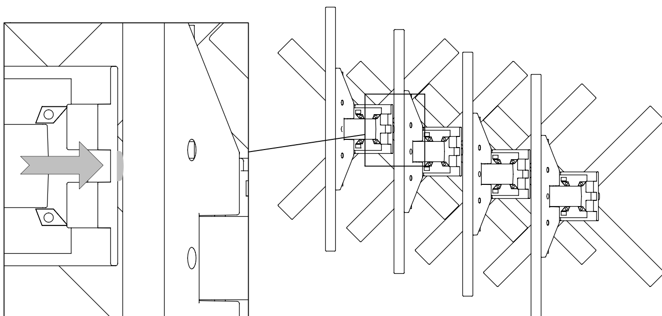
Top view Draufsicht Vue du dessus
