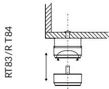
VERSTELGLEITER- ERSATZSET
