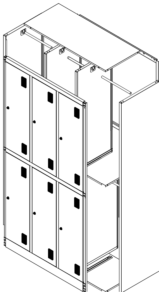
Right Side:1Pc
