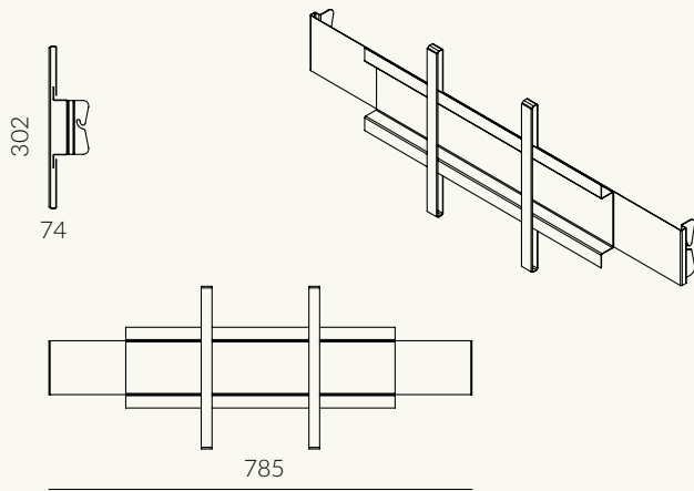
TV-holder
